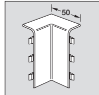
Внутренний уголок
