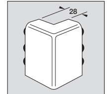
Внешний уголок
