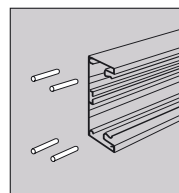
Соединительные штифты
