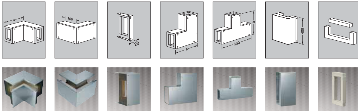
Inneneck Außeneck Endstück Flachwinkel T-Stück Schiebemuffe Versatzstück
