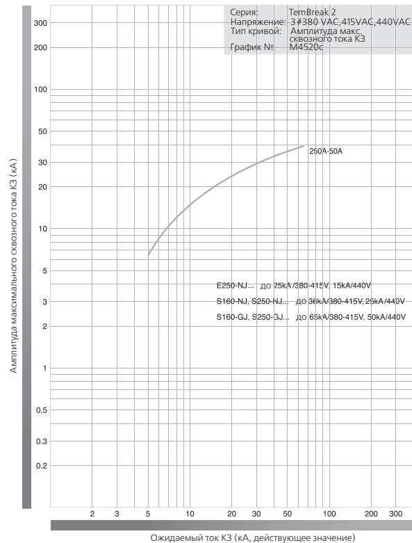
160-NJ, S160-GJ, E250-NJ, S250-NJ, 1250-GJ. 440V AC.
