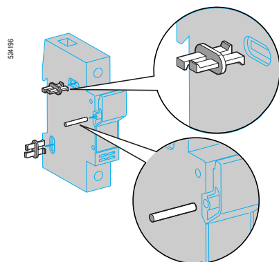
Фрагмент монтажа сборочных зажимов и шплинта
