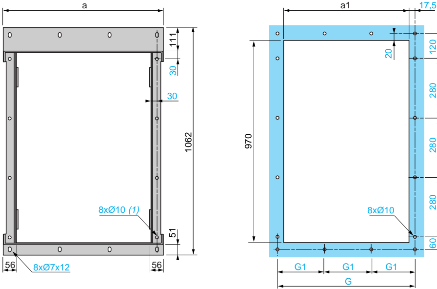
Разметка для вырезания и сверления
