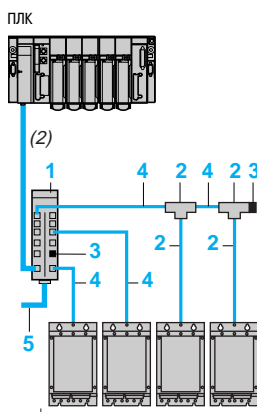
Устройства плавного пуска или ПЧ
