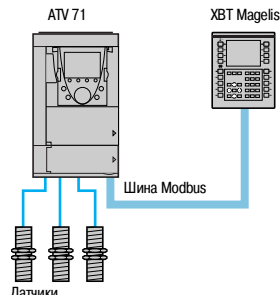
Локальный механизм с прямым подключением датчиков
