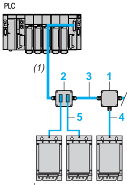
Устройства плавного пуска или ПЧ
