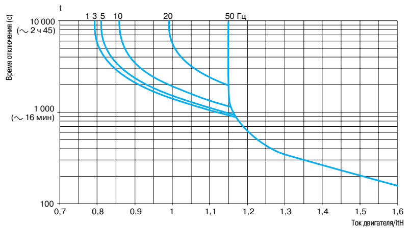
Время-токовые характеристики двигателя
