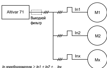
I_n преобразователя > I_{n1} + I_{n2} + \dots + I_{nx} Параллельное подключение двигателей
