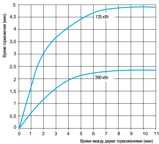
W3 A7 212 (Тормозная постоянная мощность = 200 кВт)
