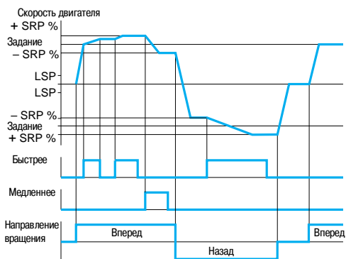
Пример обработки команд "быстрее-медленнее" вокруг заданного значения при двухпроводном управлении
